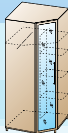
ШК-113 Шкаф 2172x891x891
