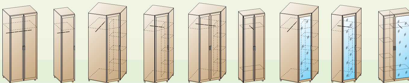
ШК-802 Шкаф 2172x896x580 ШК-803 Шкаф 2172x448x580 ШК-804 Шкаф 2172x891x891 ШК-805 Шкаф 2172x670x670 ШК-806 Шкаф 2172x856x856 ШК-808 Шкаф 2172x712x355 ШК-813 Шкаф 2172x891x891 ШК-814 Шкаф 2172x670x670 ШК-815 Шкаф 2172x896x355
