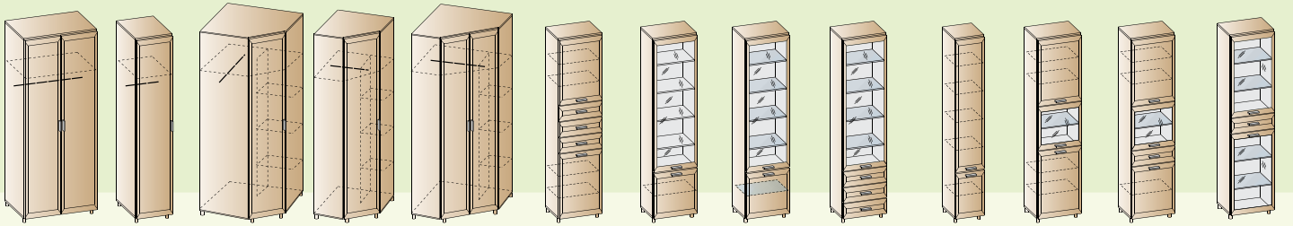
ШК-802 Шкаф 2172x896x580 ШК-803 Шкаф 2172x448x580 ШК-804 Шкаф 2172x891x891 ШК-805 Шкаф 2172x670x670 ШК-806 Шкаф 2172x856x856 ШК-807 Шкаф 2172x540x355 ШК-809 Шкаф 2172x540x355 ШК-810 Шкаф 2172x540x355 ШК-811 Шкаф 2172x540x355 ШК-812 Шкаф 2172x356x355 ШК-816 Шкаф 2172x540x355 ШК-817 Шкаф 2172x540x355 ШК-818 Шкаф 2172x540x355
