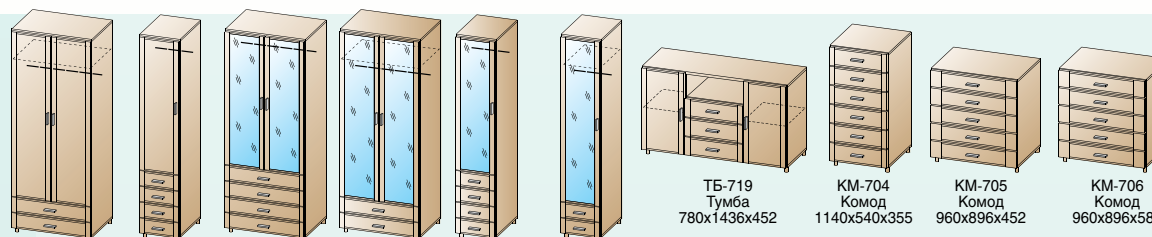
ШК-743 Шкаф 2172x896x580 ШК-744 Шкаф 2172x448x580 ШК-745 Шкаф 2172x896x580 ШК-746 Шкаф 2172x896x580 ШК-747 Шкаф 2172x448x580 ШК-748 Шкаф 2172x448x580 ТБ-719 Тумба 780x1436x452 КМ-704 Комод 1140x540x355 КМ-705 Комод 960x896x452 КМ-706 Комод 960x896x580
