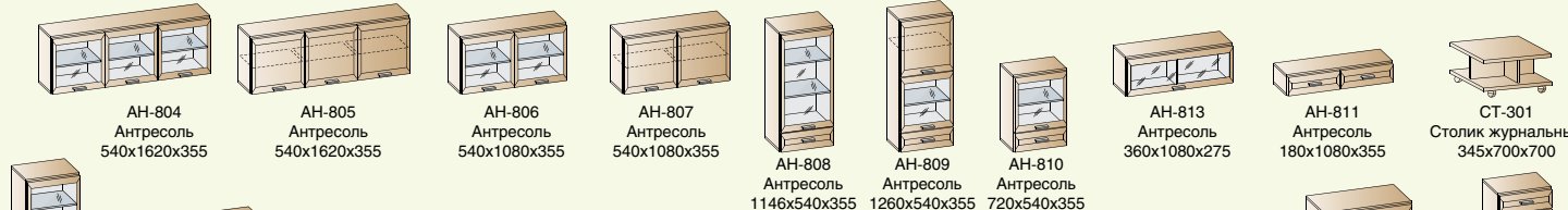
АН-804 Антресоль 540x1620x355 АН-805 Антресоль 540x1620x355 АН-806 Антресоль 540x1080x355 АН-807 Антресоль 540x1080x355 АН-808 Антресоль 1146x540x355 АН-809 Антресоль 1260x540x355 АН-810 Антресоль 720x540x355 АН-813 Антресоль 360x1080x275 АН-811 Антресоль 180x1080x355 СТ-301 Столик журнальный 345x700x700 ТБ-801 Тумба 1320x540x355 ТБ-819 Тумба 780x1436x452 ТБ-803 Тумба 600x540x355 ТБ-804 Тумба 600x1080x355 ТБ-805 Тумба 420x1080x530 ТБ-806 Тумба 420x1620x530 ТБ-807 Тумба 420x1080x530 ТБ-808 Тумба 420x540x530 ТБ-825 Тумба 600x540x355 КМ-805 Комод 960x896x452 КМ-804 Комод 1140x540x355
